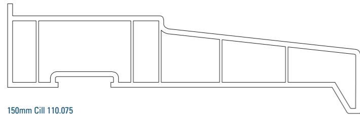
150mm Cill 110.075
